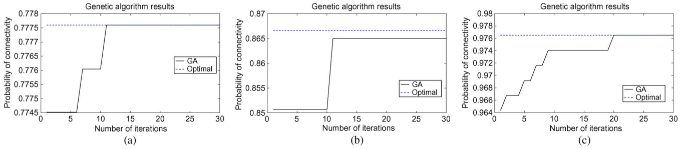
Fig. 16. GA scenarios. (a) Scenario 1. (b) Scenario 2. (c) Scenario 3.
